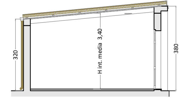
SEZIONE A-A
